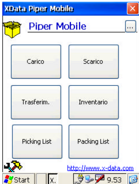
Finestra principale
